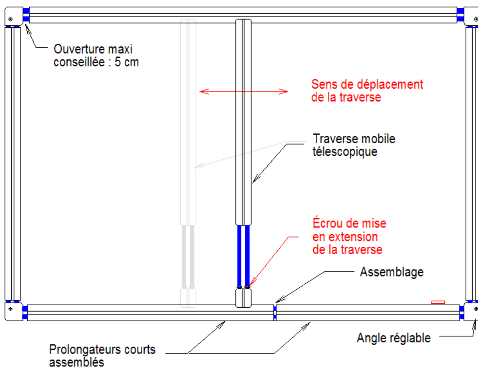
Fig. 1 : Plan du bâti
