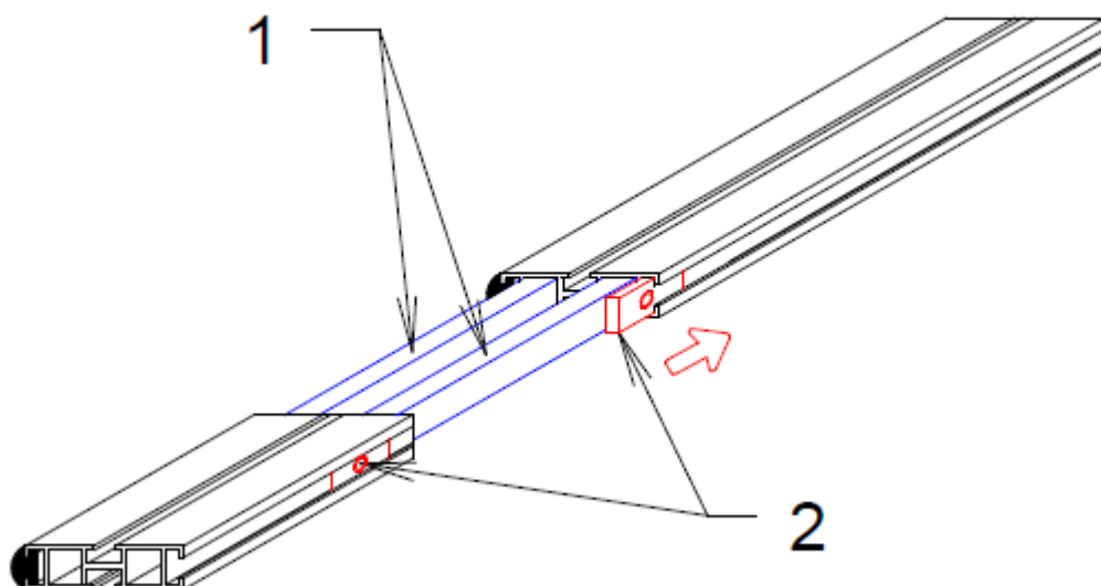
Fig. 3 : Mode opératoire
