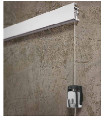
Rail R20 – 23 × 11,7 mm, charge jusqu'à 30 kg. Pour utilisation avec des tringles, veiller à laisser un espace entre le rail et le plafond.
