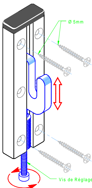
Modèle standard: Fixation par 6 vis à bois
