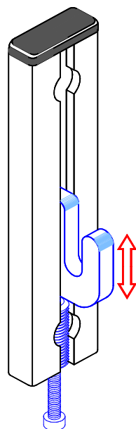
Fixation pour 2 chevilles chimiques
