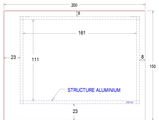
Plateau standard : vue de dessus
