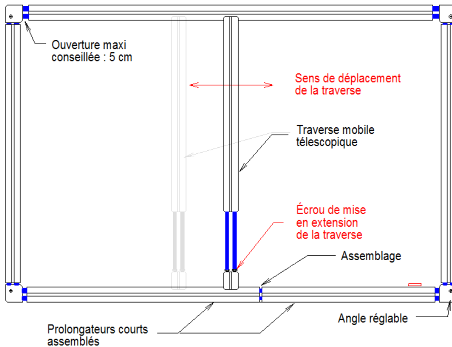
Fig. 1 : Plan du bâti
